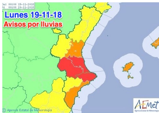
Avisos por lluvias para el día 19-11-18 (Fuente: AEMET)
