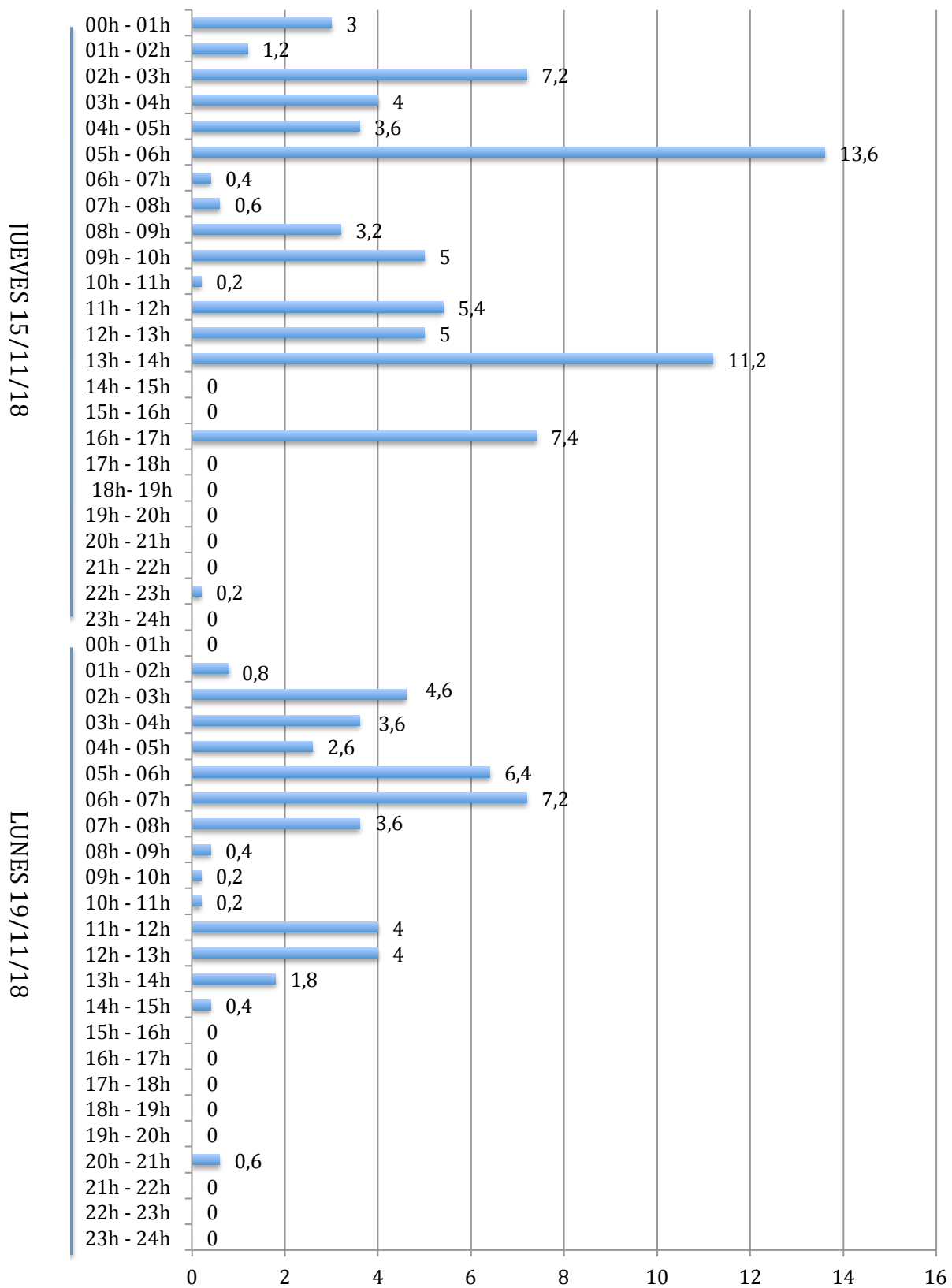
Cantidades de lluvia registradas por horas en ALBERIC (estación Zona San Cristóbal) los días 15 y 19/11/18 (en l/m²)
