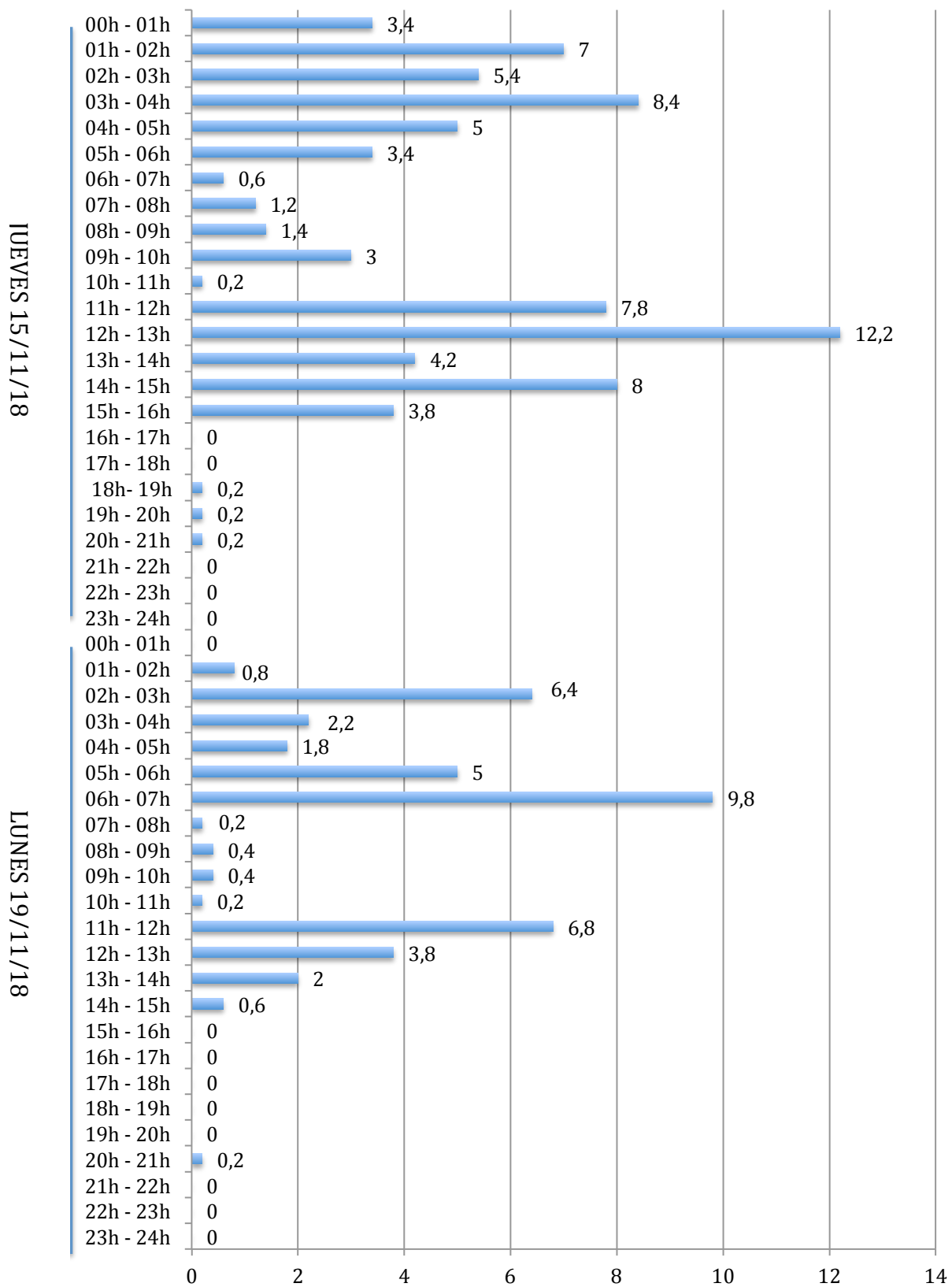
Cantidades de lluvia registradas por horas en ALBERIC (estación Ayuntamiento) los días 15 y 19/11/18 (en l/m²)
